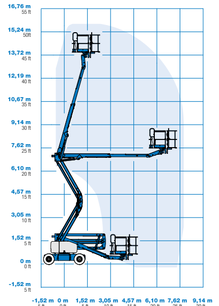
Courbe de travail Z-45/25
