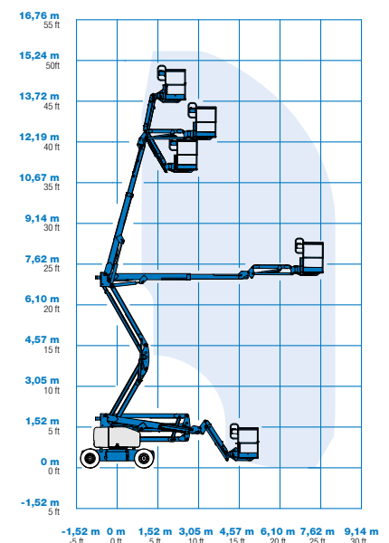
Courbe de travail Z-45/25J
